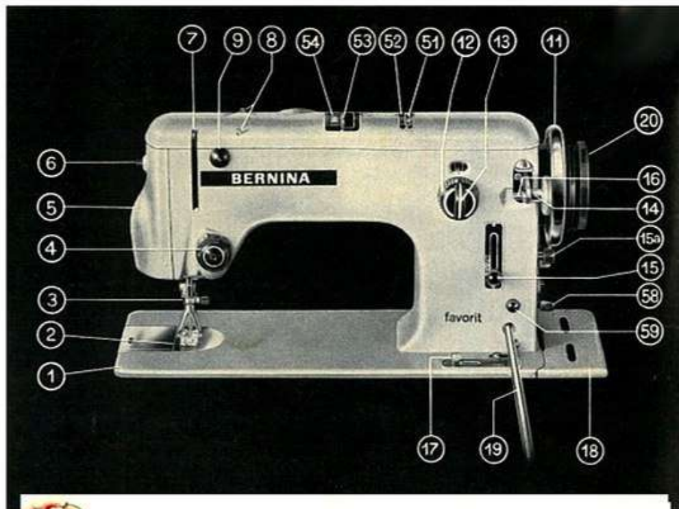
In der nebenstehenden Fig. 1 ist eine BERNINA-Favorit Kl. 540-1 (Zickzacknähmaschine mit Zierstich-Automatik) mit Horizontalmotor dargestellt, unter namentlicher Kennzeichnung der Bedienungseinrichtungen usw., deren Bezeichnungen in der Gebrauchsanleitung angewendet werden.
