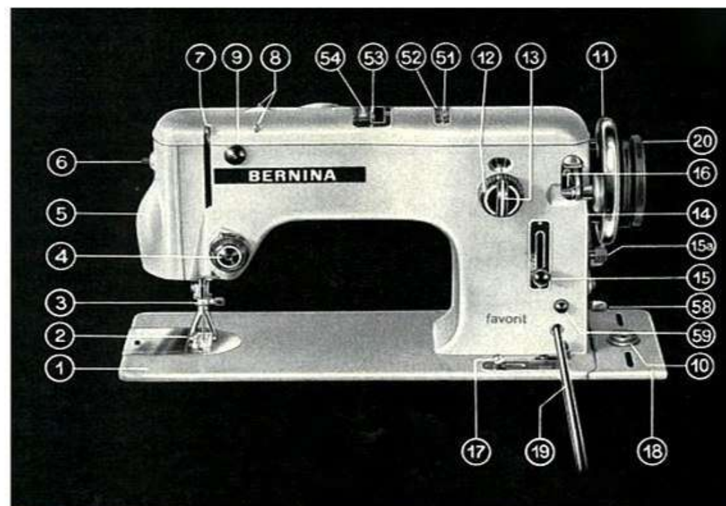
In der nebenstehenden Fig. 2 ist eine BERNINA-Favorit Kl. 540-1 (Zickzacknähmaschine mit Zierstich-Automatik) für Treteinrichtung dargestellt, unter namentlicher Kennzeichnung der Bedienungseinrichtungen usw., deren Bezeichnungen in der Gebrauchsanleitung angewendet werden.
